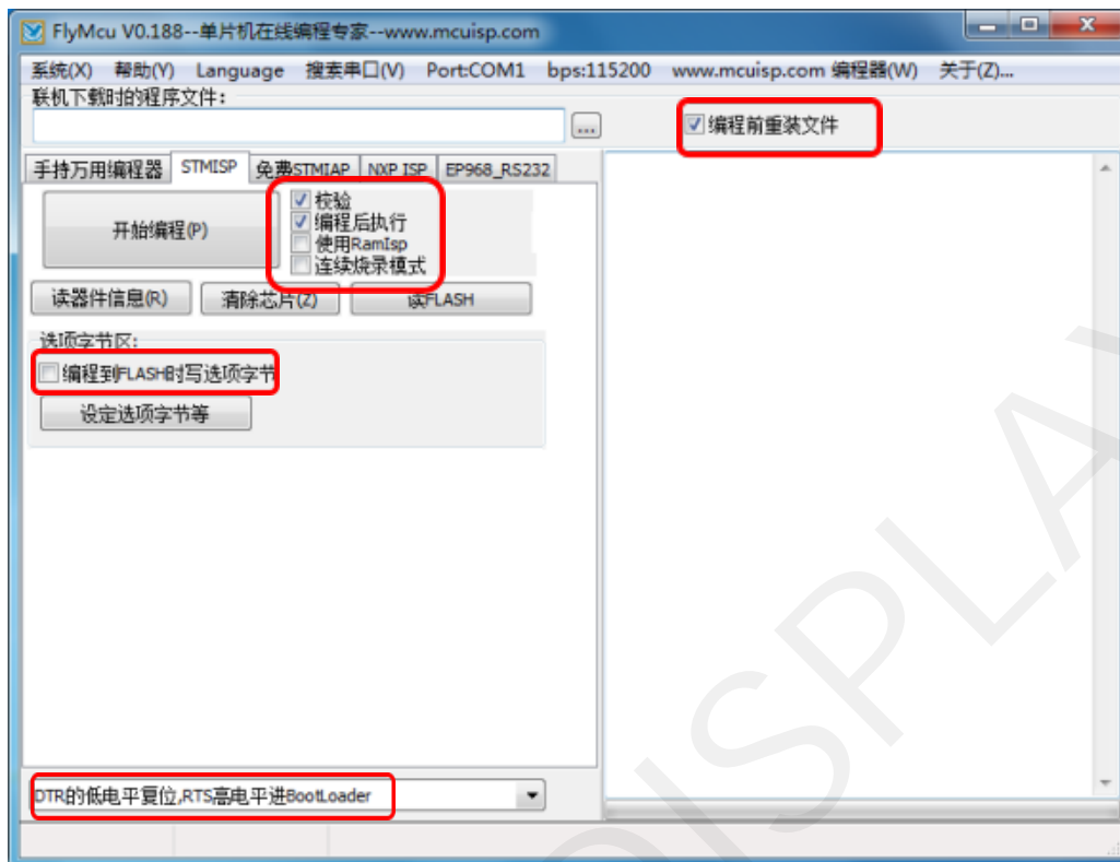
图 12 lyMcu 配置
