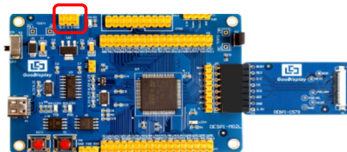
图 11 P12 短接位置
